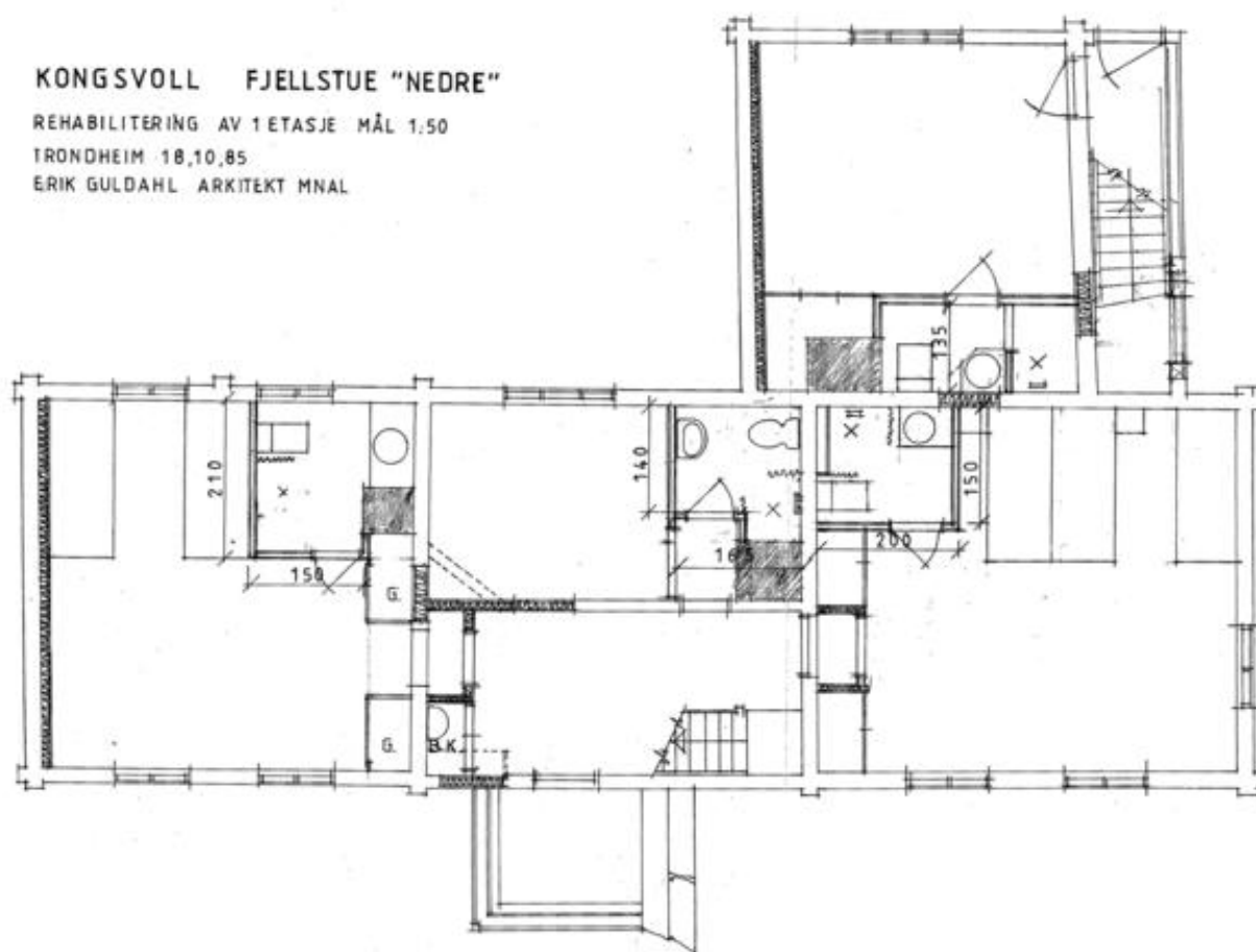
Plan 1. etasje.
