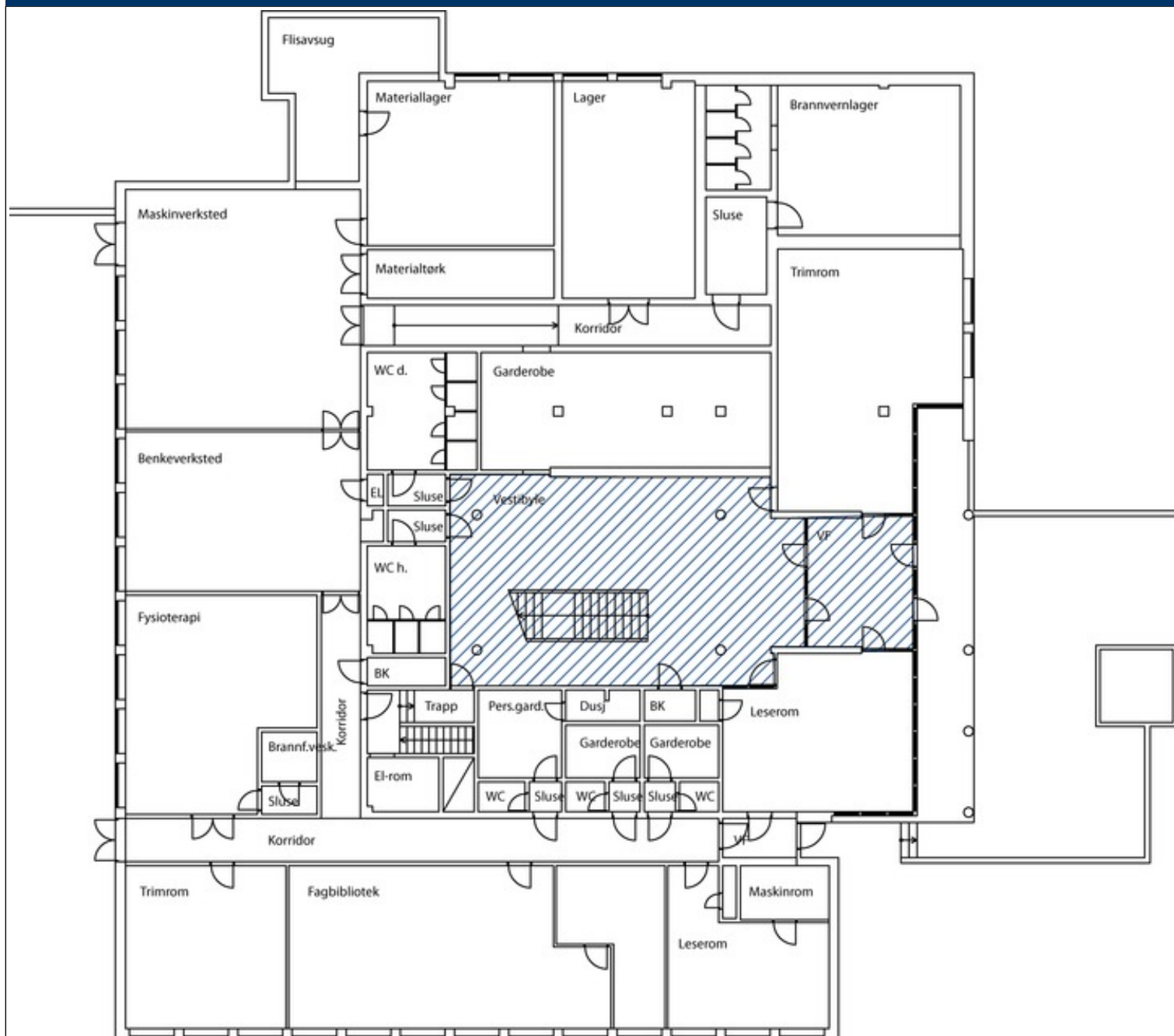
Plantegning underetasje, G10. Omfang interiørfredning er markert med blå skravur.
