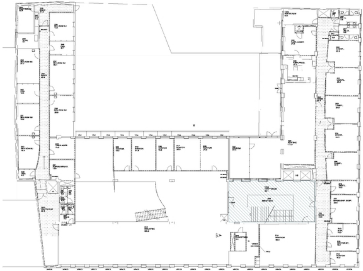
Plantegning 2. etasje. Omfang interiørfredning er markert med blå skravur. Opphavsrett: Statsbygg.
