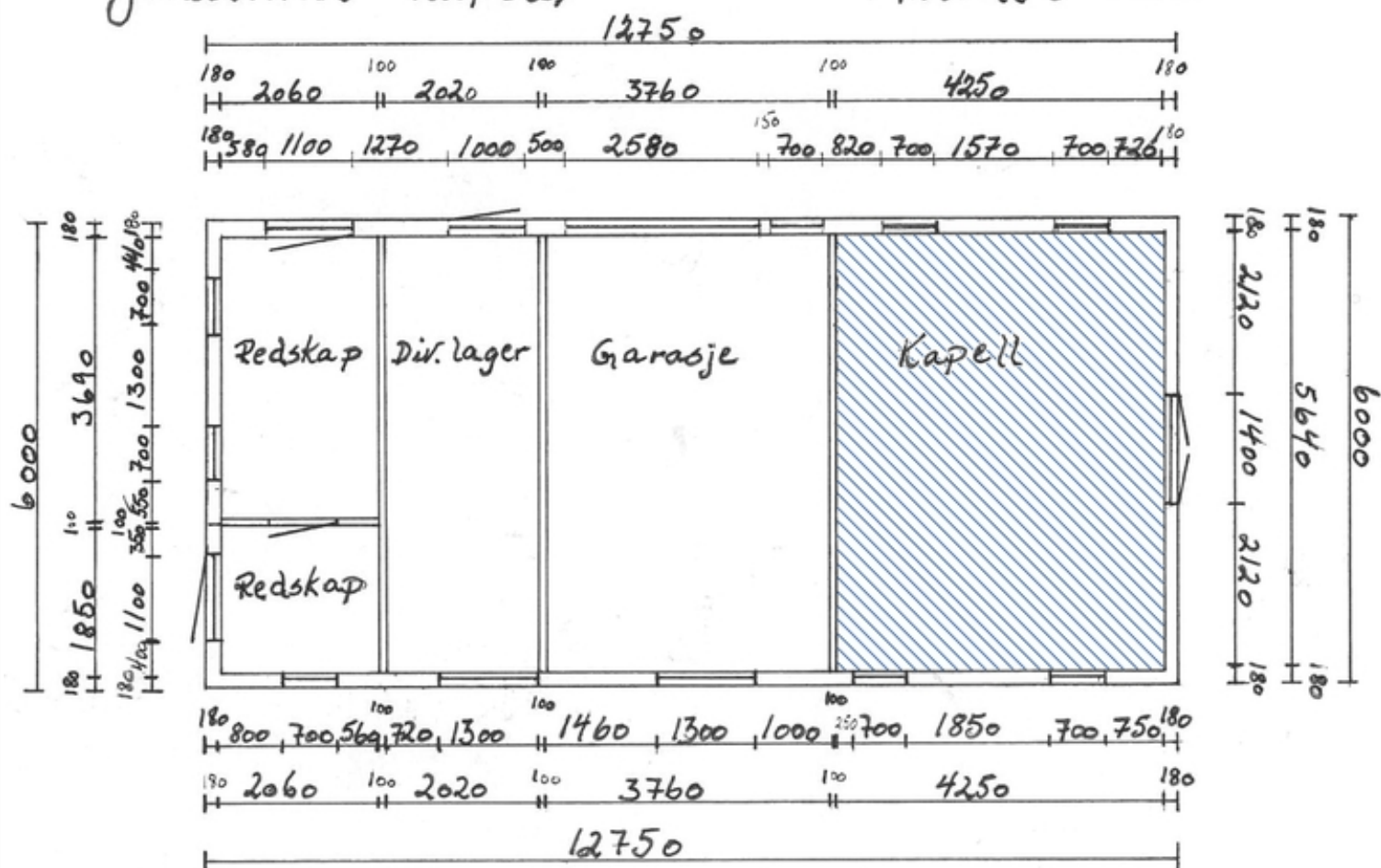
Plantegning 1. etasje, kapell. Omfang interiørfredning er markert med blå skravur.
