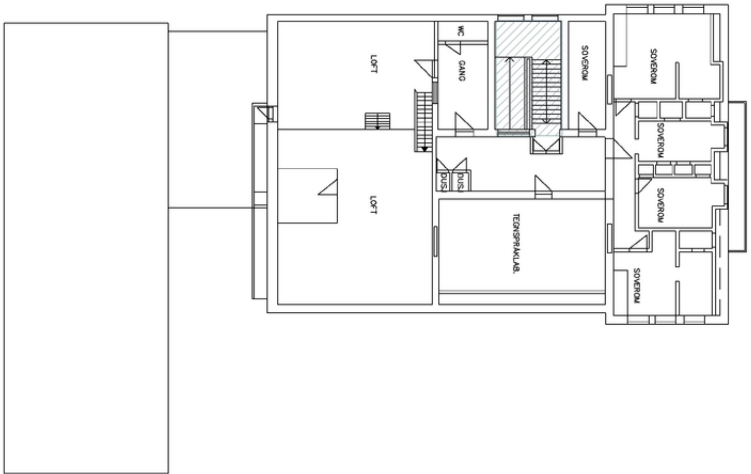
Plantegning 3. etasje. Omfang interiørfredning er markert med blå skravur. Opphavsrett: Statsbygg.
