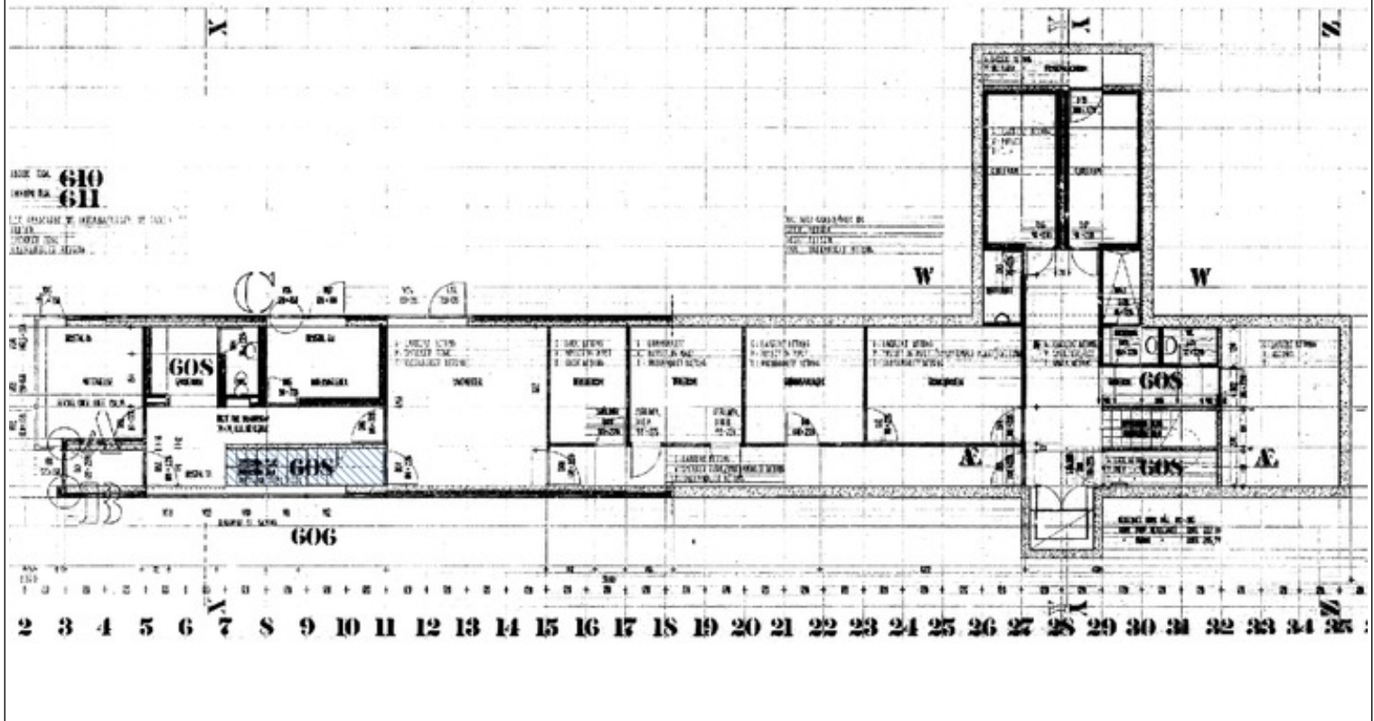
Plantegning kjeller. Omfang interiørfredning er markert med blå skraver.
