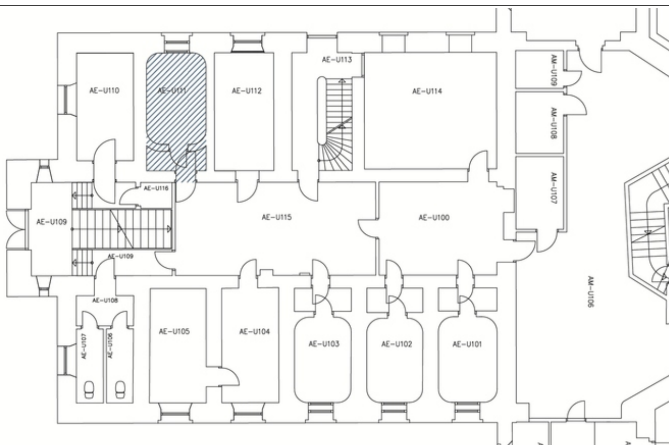
Plantegning kjeller Blokk E. Omfang interiørfredning er markert med blå skraver.
