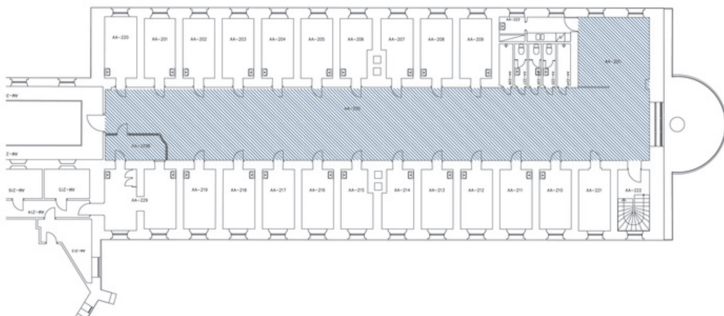
Plantegning 2. etasje Blokk A. Omfang interiørfredning er markert med blå skraver.
