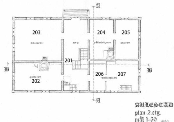
Grunnplan 2. etasje.
