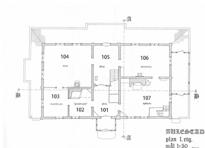
Grunnplan 1. etasje.
