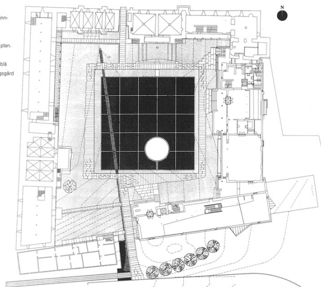
Plantegning ca. 1997. Opphavsrett: Etter Byggekunst nr. 2 1998.
