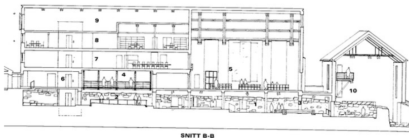
Tverrsnitt som også viser sammenheng mellom utstillingsarealer i ringmuretasjen i Bispefløyen og Museet. Opphavsrett: Etter Statsbygg ferdigmelding 526/1997.
