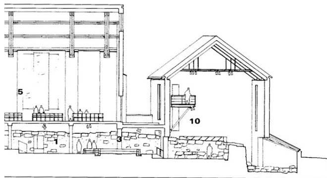
Tverrsnitt gjennom østre del som også viser forbindelsen til utstillingen i ringmuretasjen i Bispefløyen. Opphavsrett: Etter Statsbygg ferdigmelding 526/1997.
