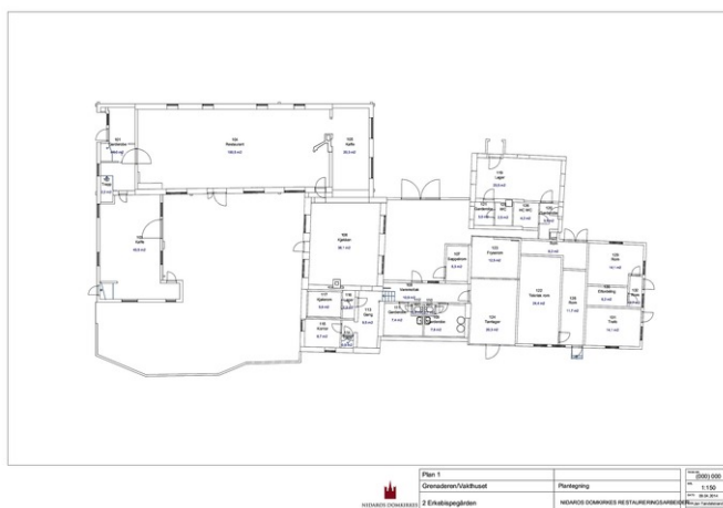
Grunnplan 1. etasje. Opphavsrett: NDR.
