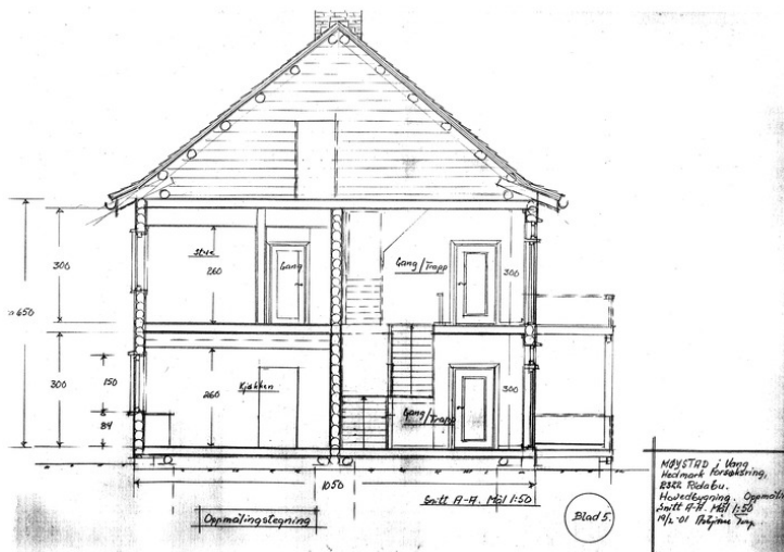
Snitt, oppmåling 2001.
