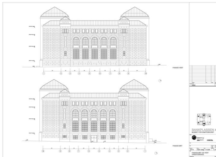
Fasader mot øst og vest. Opphavsrett: Statsbygg.
