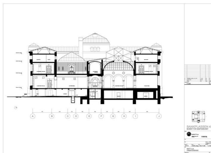
Snitt. Opphavsrett: Statsbygg.
