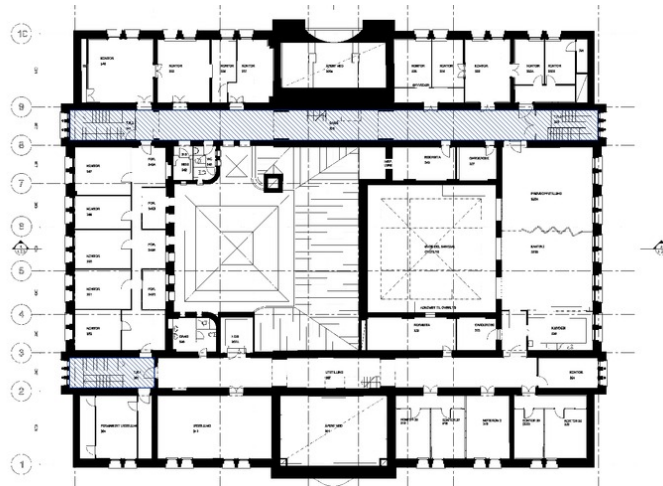
Plan 3. etasje. Fredet interiør er skravert.
