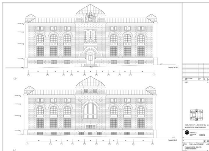
Fasader mot nord og syd. Opphavsrett: Statsbygg.
