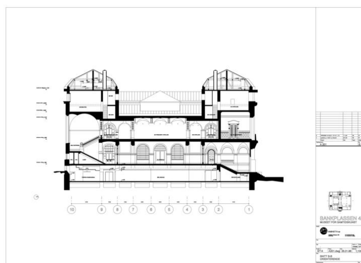
Snitt med hovedinngangen fra Bankplassen til høyre. Opphavsrett: Statsbygg.
