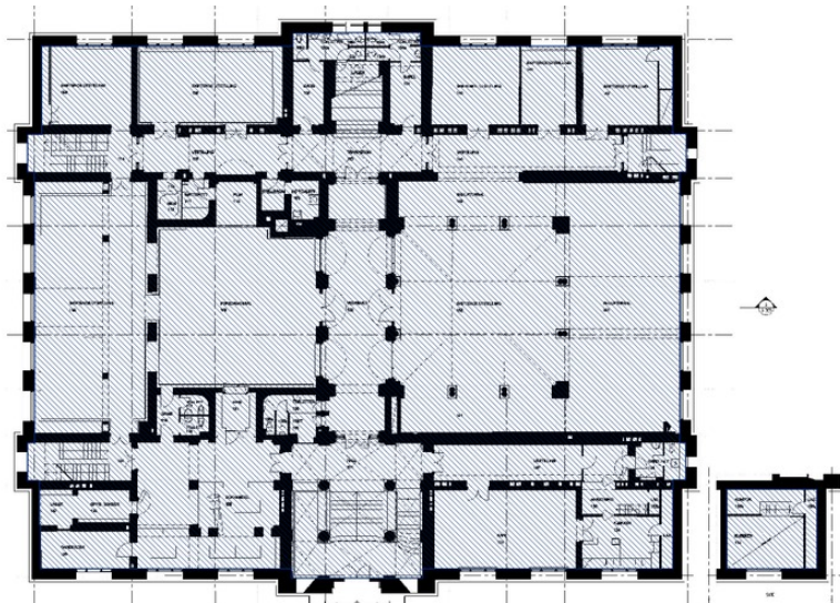
Plan 1. etasje. Interiøret i hele etasjen er fredet.
