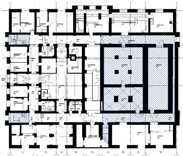
Plan kjeller. Fredet interiør er skravert.
