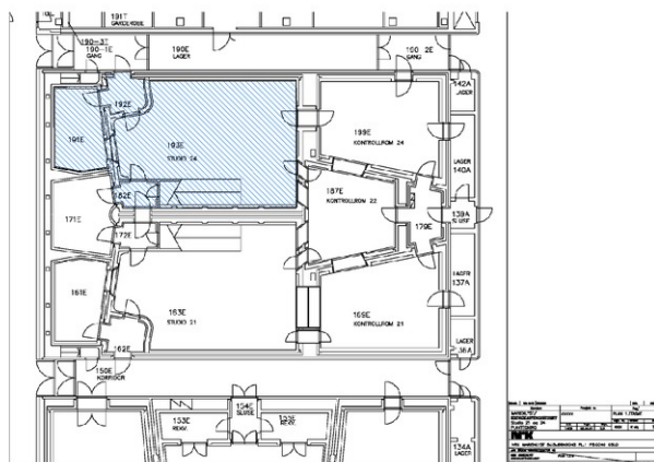
Hørespillstudio. Fredet interiør er skravert og dekker arelaet 182 E, 191 E, 192 E og 193 E.
