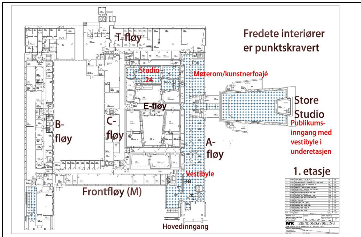
Plantegning, 1. etasje. Rom med fredet løst inventar markert med rødt.
