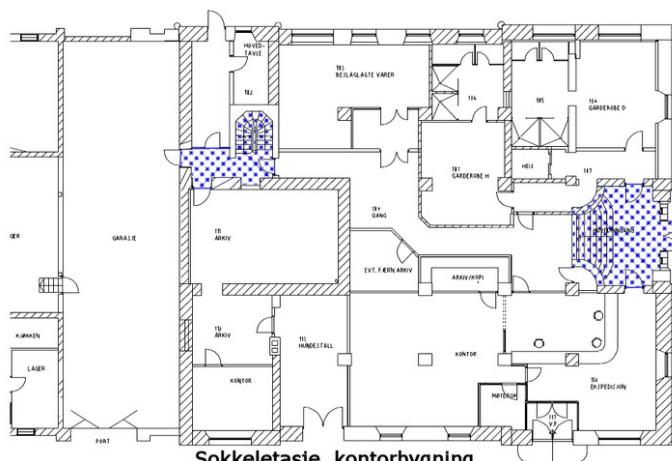
Sokkeletasje, kontorbygning Fredete interiører er punktskravert
