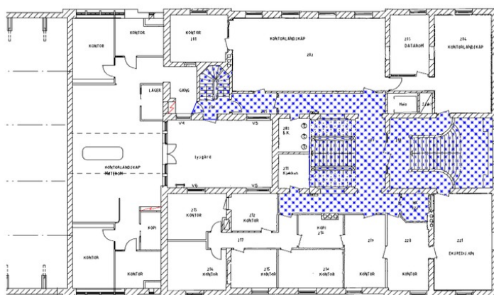
1. etasje, kontorbygning Fredete interiører er punktskravert
