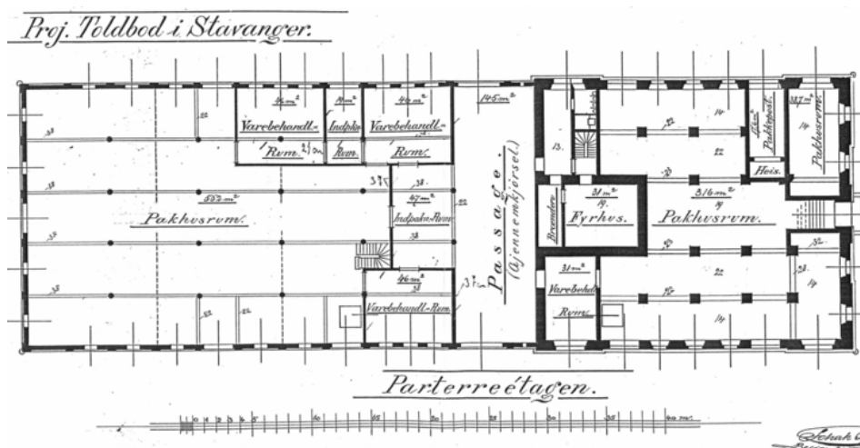
Oppr. inndeling i nederste etasje i hoved- og pakkehusfløy med pakkehus- og varebehandlingsrom. Opphavsrett: Schak Bull 1903. Etter kopi i Riksantikvarens arkiv.
