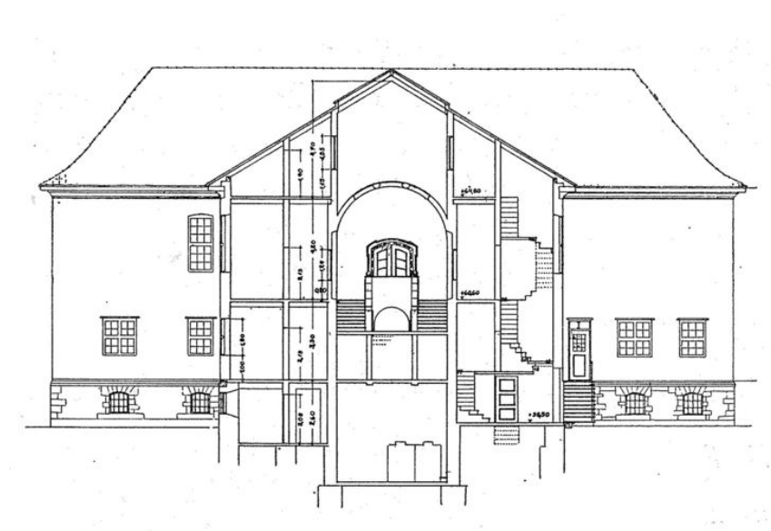
Tverrsnitt etter Byggekunst 1924.
