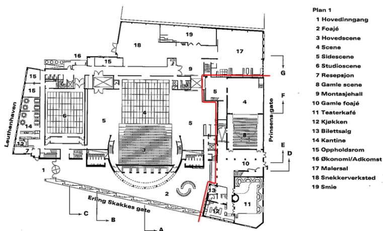
Plan 1. et. Fredningen omfatter alle deler som eksisterte ved fredningsvedtaket i 1969, her avgrenset med rødt i 2008. Opphavsrett: Planunderlag: Statsbygg, etter ferdigmelding 1997.
