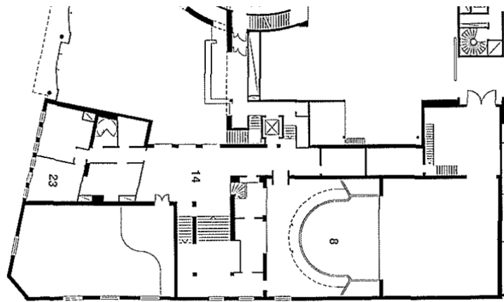
Plan 2. et. Nord er t.h. på tegningen. Etter Byggekunst 1998.
