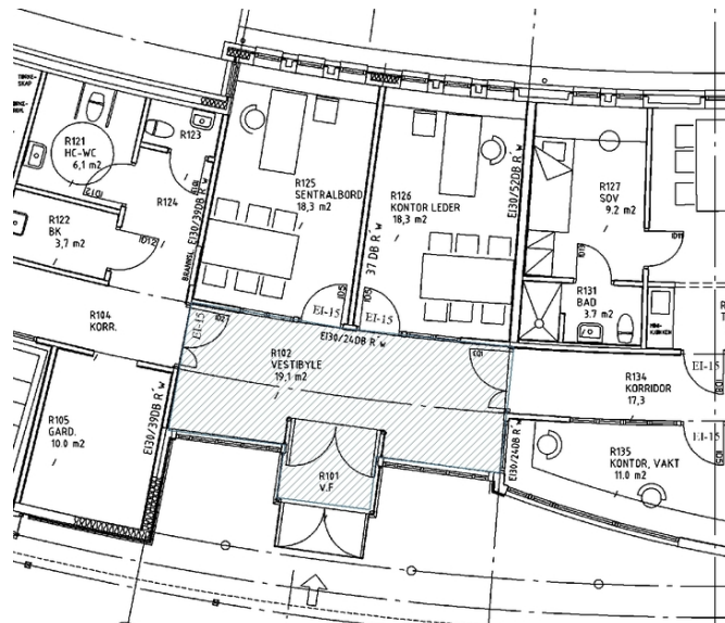
Utsnitt av plantegning 1. etasje med skravur for fredet interiør. Opphavsrett: Statsbygg.
