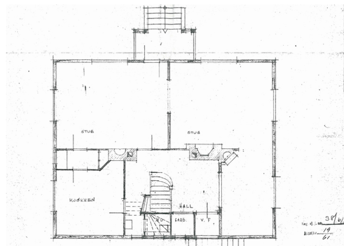
Oppmålingstegning av 1 etg datert 20.3.1960. Opphavsrett: Statsbygg.
