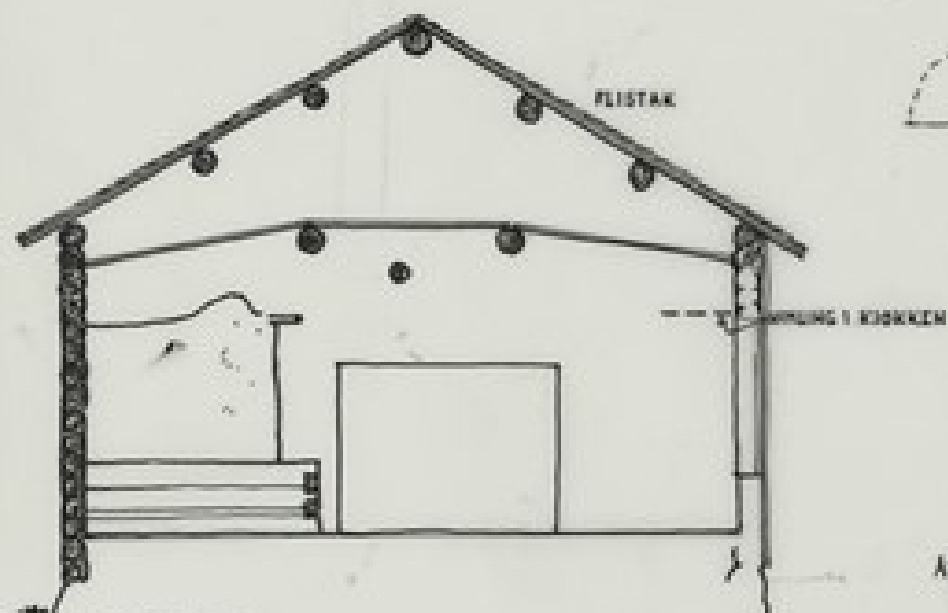
SNITT A-A
