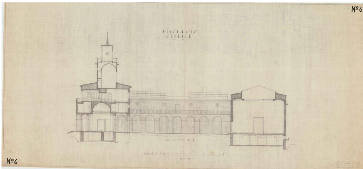
Snitt øst – vest gjennom hovedinngang med tårn, midtgård samt bakre fløy mot Solheimgaten.
