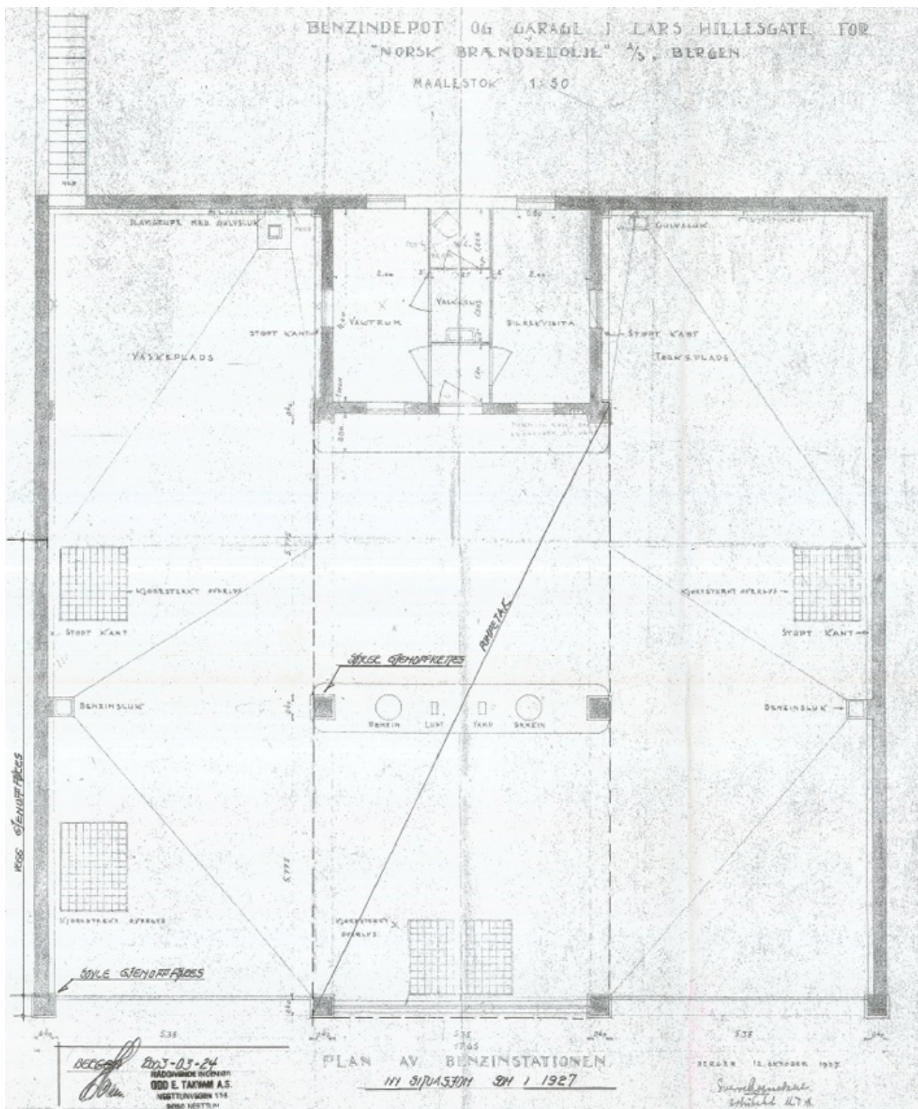
Grunnplan av stasjonen slik han vart planlagt, med tilbakeføringer frå siste restaurering avmerka. Planløysinga i ekspedisjonslokalet er i dag ei anna, med eitt stort rom framme og tre små rom i bakkant, og vart kanskje aldri utført som på denne teikninga. Byggesaksarkivet, Bergen kommune
