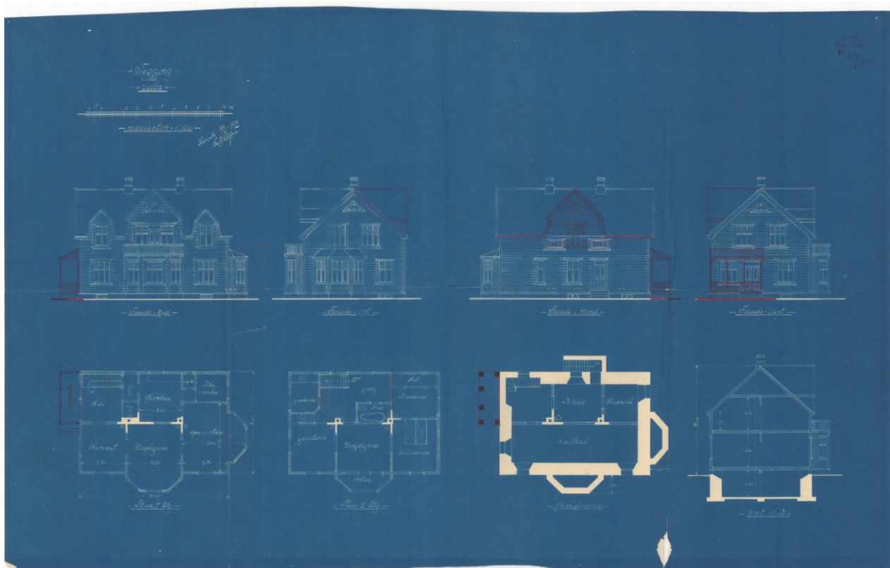
Figur 5 Byggetegninger av Sveins gate 15, 1923. Endringer fra opprinnelig søknad markert med rødt.
