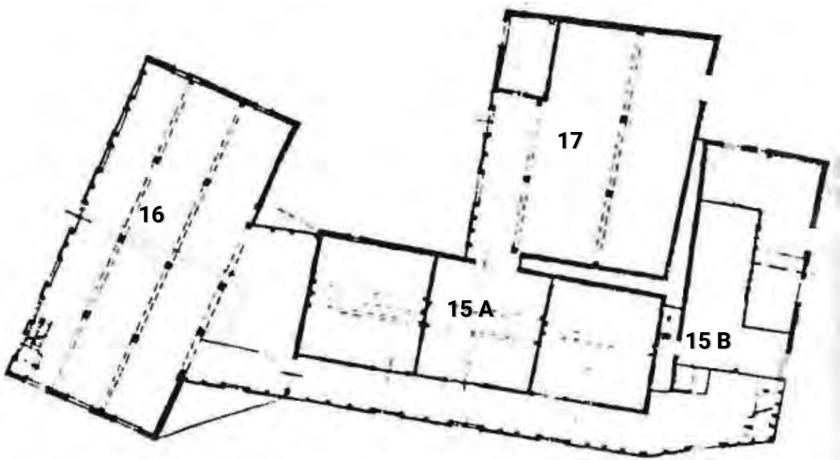
Sandviksbodene 15-17. Laftekjernane i bod 16 er fjerna og erstatta med stolpar/dragarar. Oppmålingsteikning av arkitekt Oddvin Storebø, ca. 1950.
