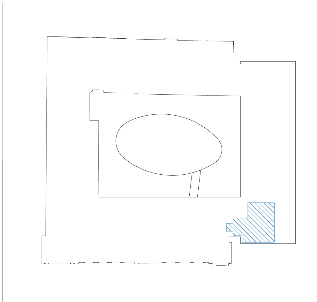
Plantegning Nordkvaralet 2. etg. Omfang interiørfredning er markert med blå skarvur. Opphavsrett: Statsbygg.
