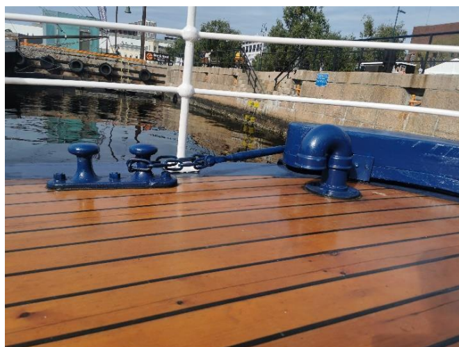
Pullere og svane-hals for lufting – BB-side.
