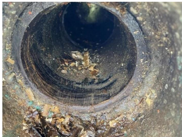
Den gamle pokkenholt-hylsa akter. Foto: Alexander Ytteborg, 16.8.2022.
