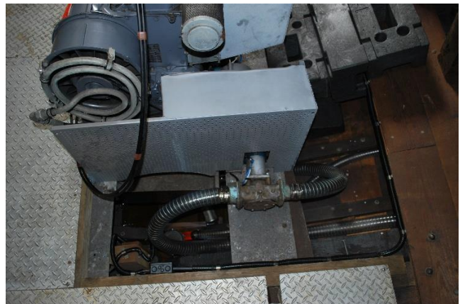
Nødlensepumpe med magnetstyrt innslag.
