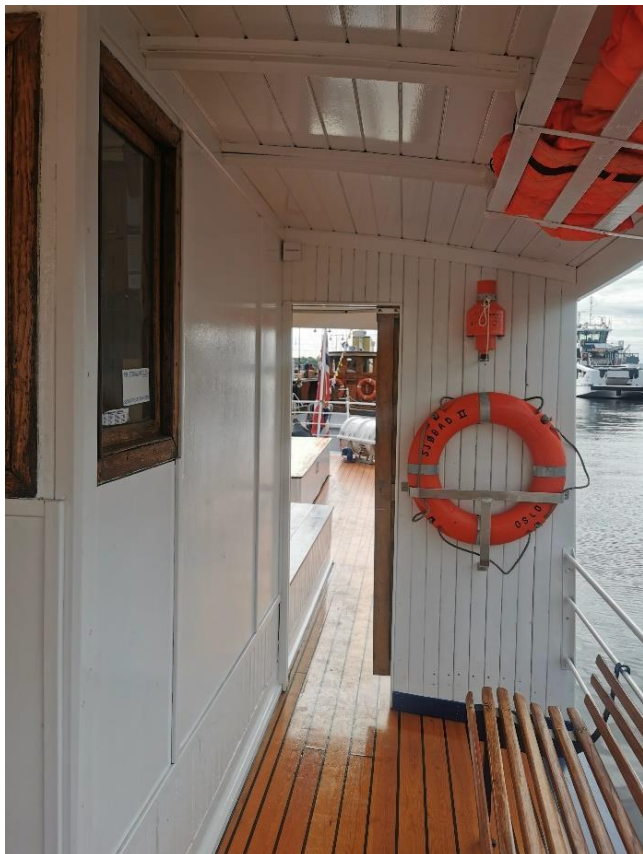
Under takoverbygg fordekk, BB-side. Legg merke til døren i skilleveggen.
