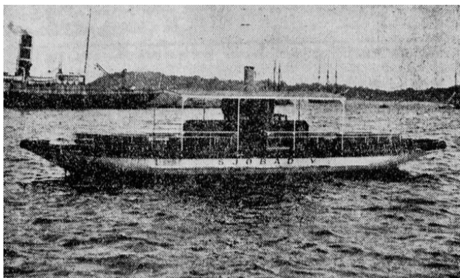
Leveransefoto av M/S «Sjøbad V».
