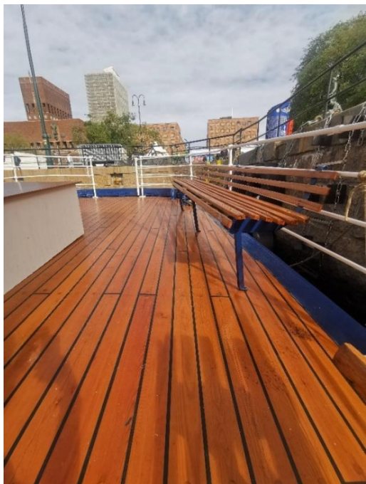
Fordekk, benker og livebelteklasse, SB side.
