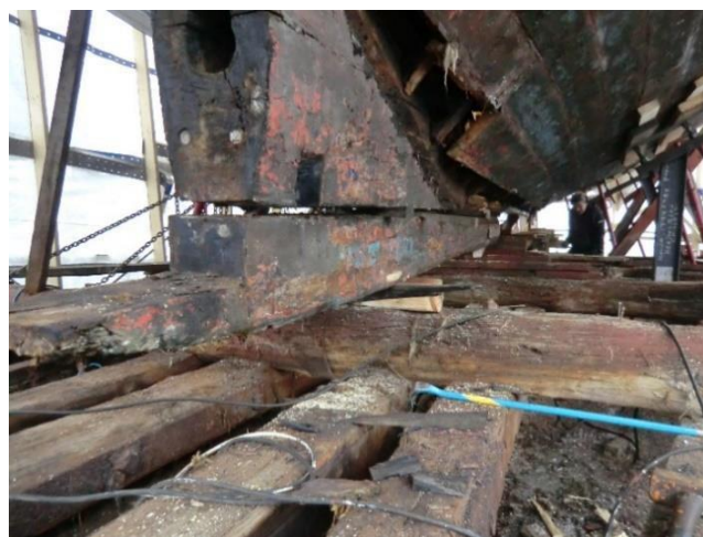
Gammel gjennomføring til propellaksling forut.
