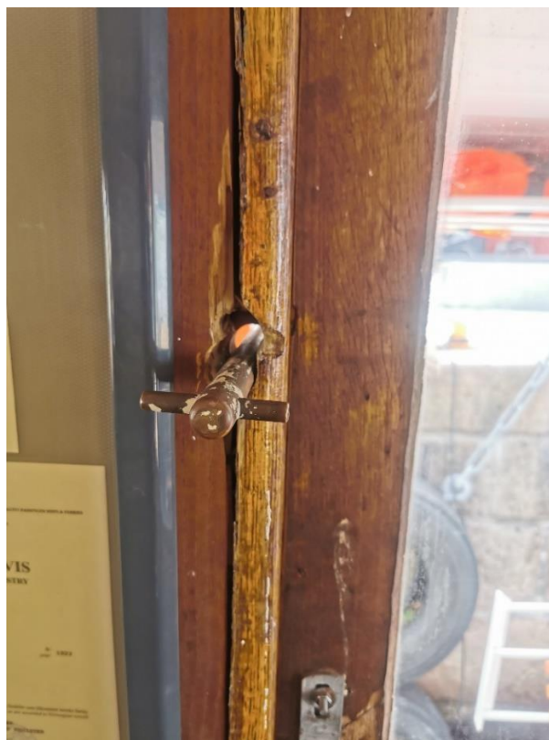
Spak til å lukke utvendig skilledør på styrbord side.
